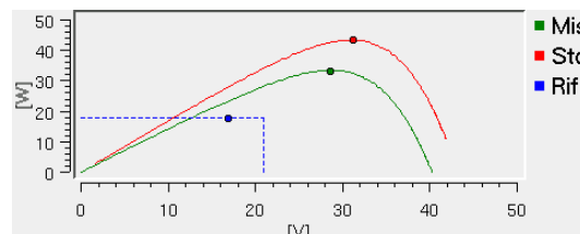
Curva caratteristica in potenza
