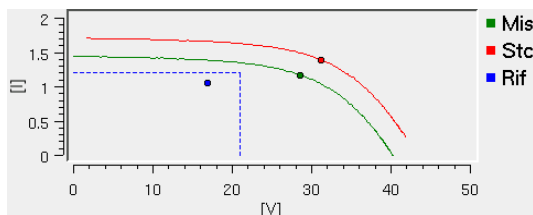
Curva caratteristica in corrente
